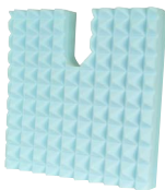
▲ COCCYX
